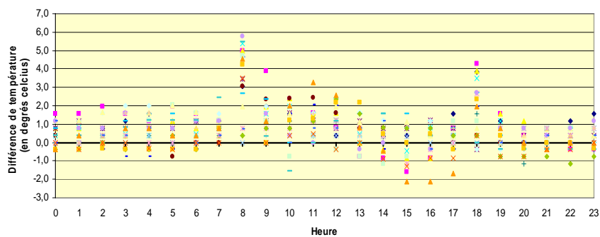
Variation de la différence de température entre l'intérieur et l'extérieur de l'abri filet heure par heure, août 2010: Ferme La Cueille
